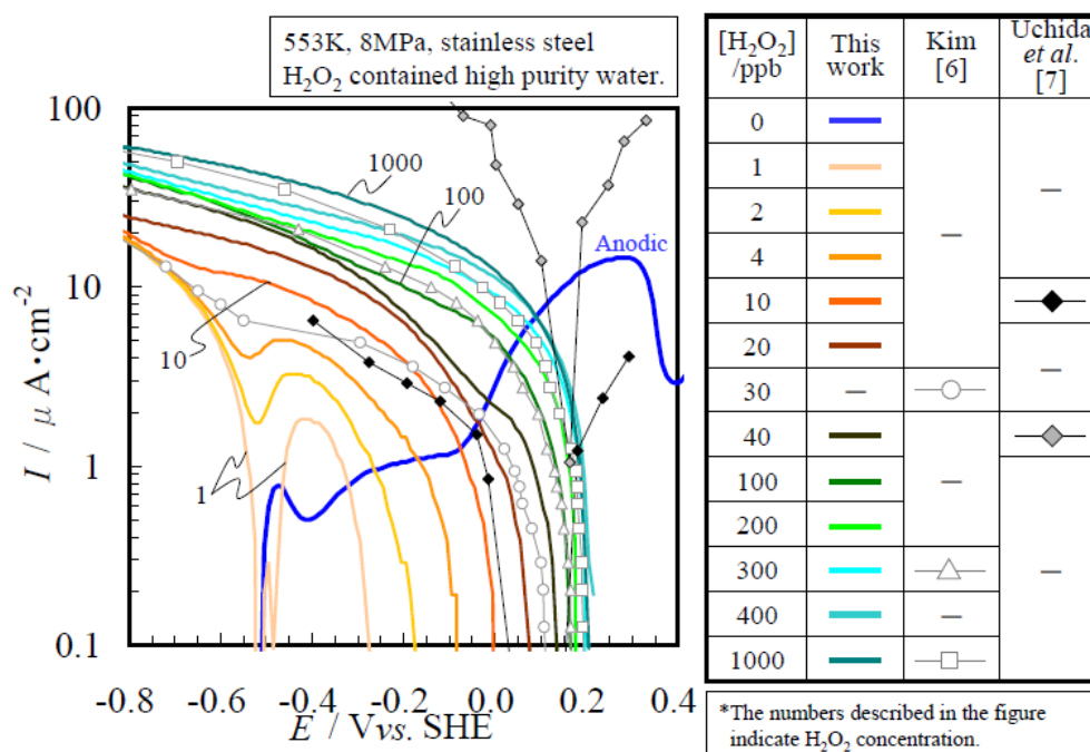
図 5.9 高温純水中の SUS316L 上での過酸化水素のカソード分極曲線の測定例 (11)
