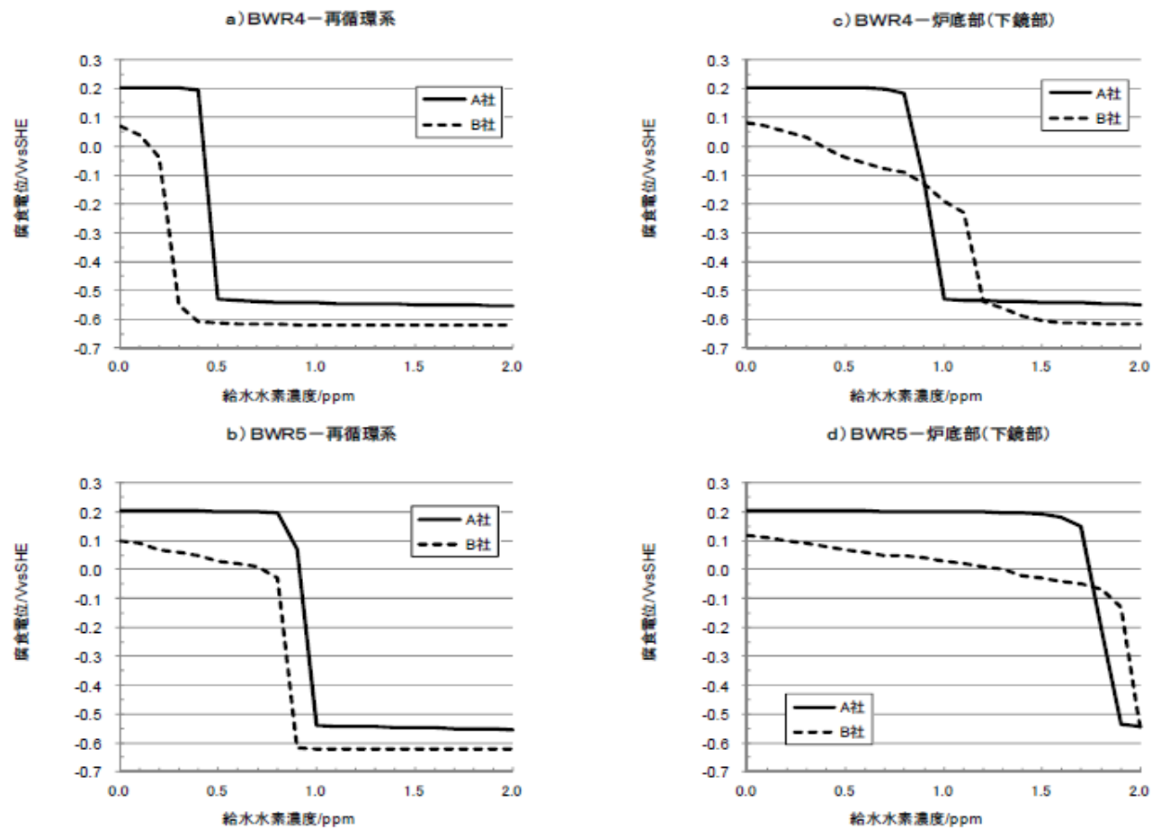
添付図 1-6 BWR-4 並びに BWR-5 での再循環系配管内面及び炉底部の腐食電位
