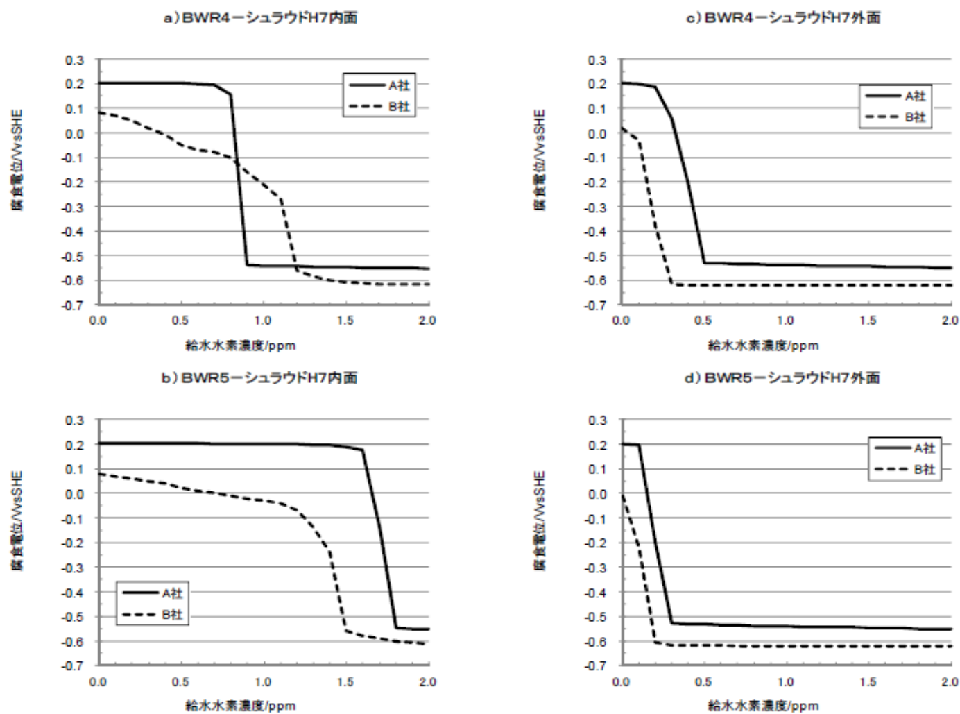
添付図 1-5 BWR-4 並びに BWR-5 でのシュラウド H7 内外面の腐食電位
