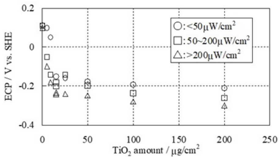
添付図 2-2 腐食電位低下に対する酸化チタン付着量依存性 (2)
