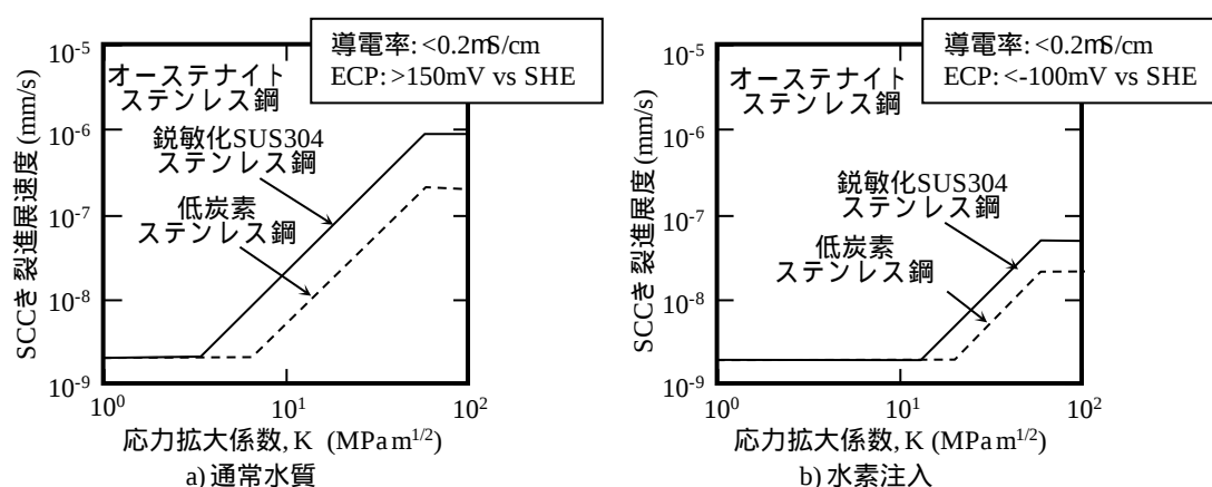
図 1.9 日本機械学会維持規格におけるき裂進展速度評価 (7)
