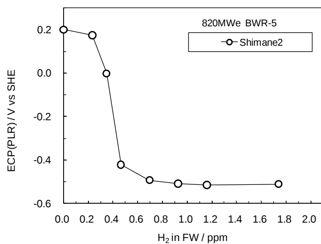
図 2.8 820MWe - BWR-5 の PLR サンプリングラインでの腐食電位実測値 (13)
