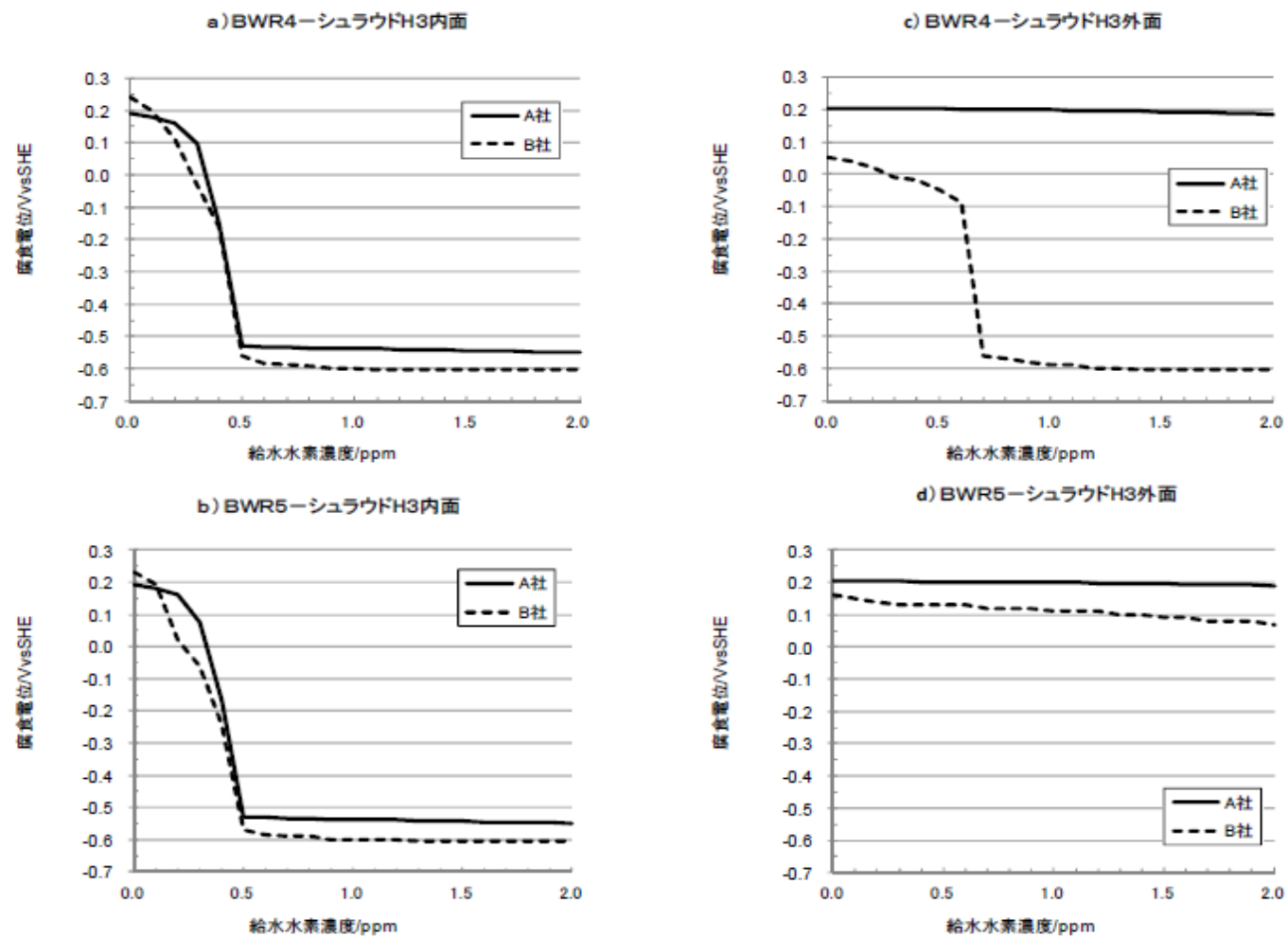
添付図 1-2 BWR-4 並びに BWR-5 でのシュラウド H3 内外面の腐食電位
