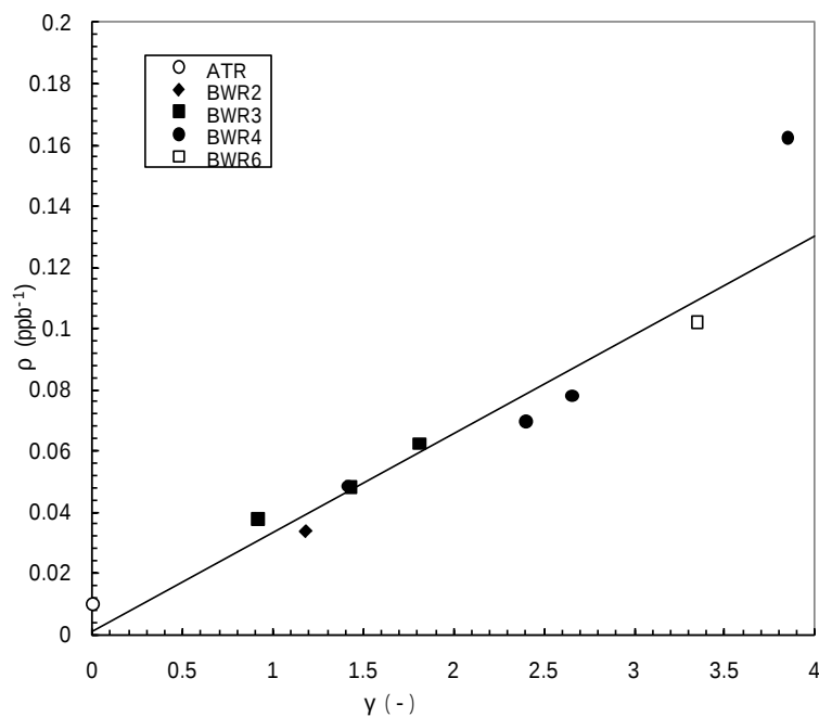
図 2.10 再循環系での再結合効率を示す \rho とダウンカマ平均線量率に関連する指標 \gamma の関係 (18)
