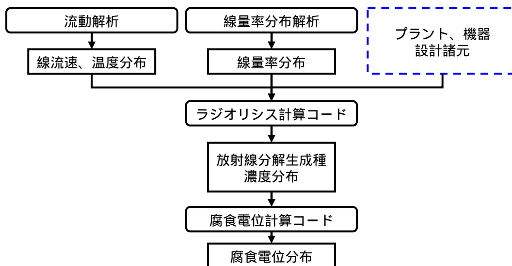
図 3.10 腐食環境評価の流れ (8)
