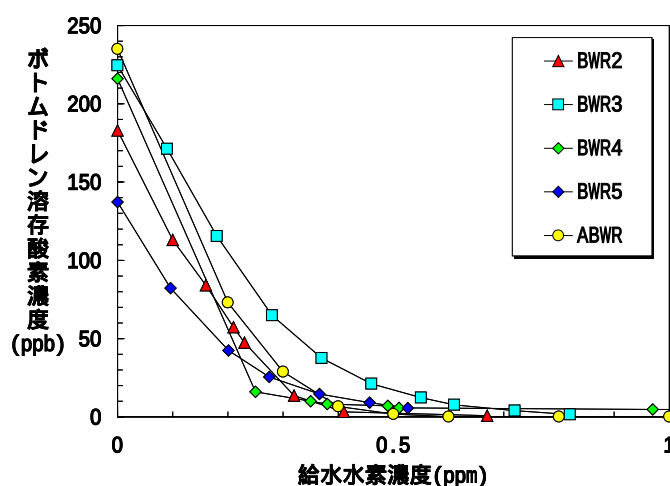
図 2.4 ボトムドレンの溶存酸素濃度と水素注入量との相関（実機での測定例） (4)
