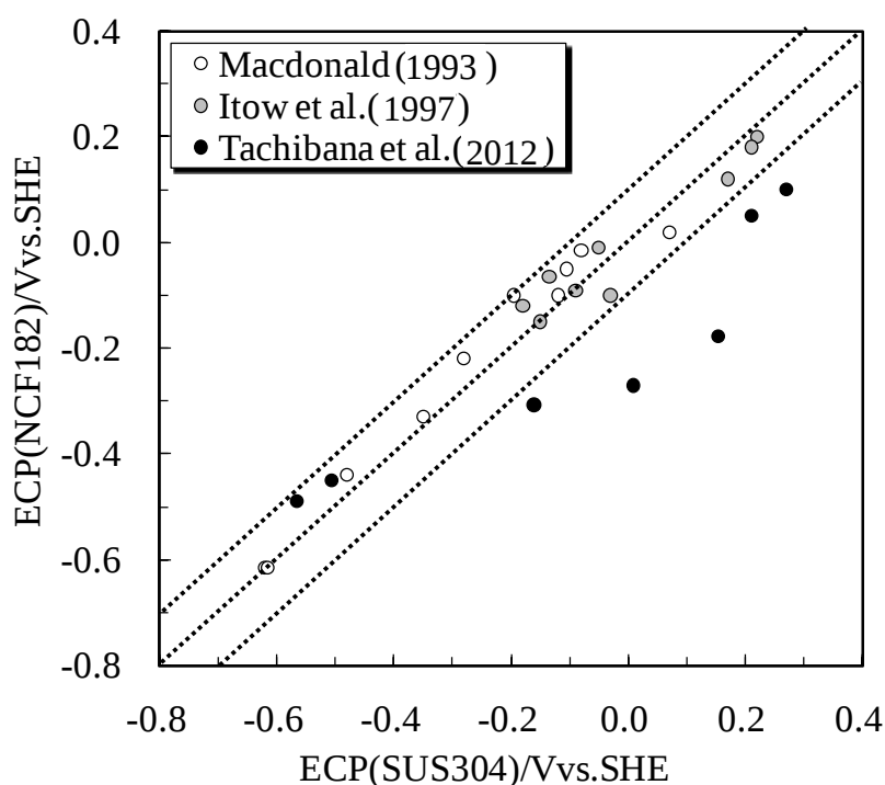
図 3.15 304 ステンレスと 182 ニッケル基合金の腐食電位の相関[参考文献 14-16 を基に作成]
