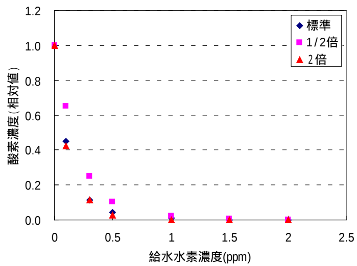
図 5.13 炉底部水質に及ぼすダウンカマ線量率の影響 (上段：過酸化水素，下段：酸素)
