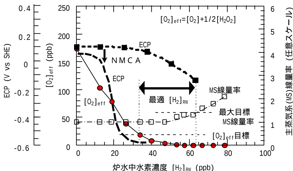
図 1.8 水素注入効果と最適水素注入量 (3)
