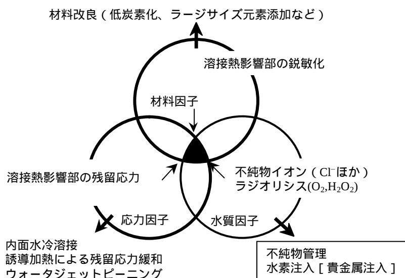
図 1.2 応力腐食割れの主要因と抑制策
