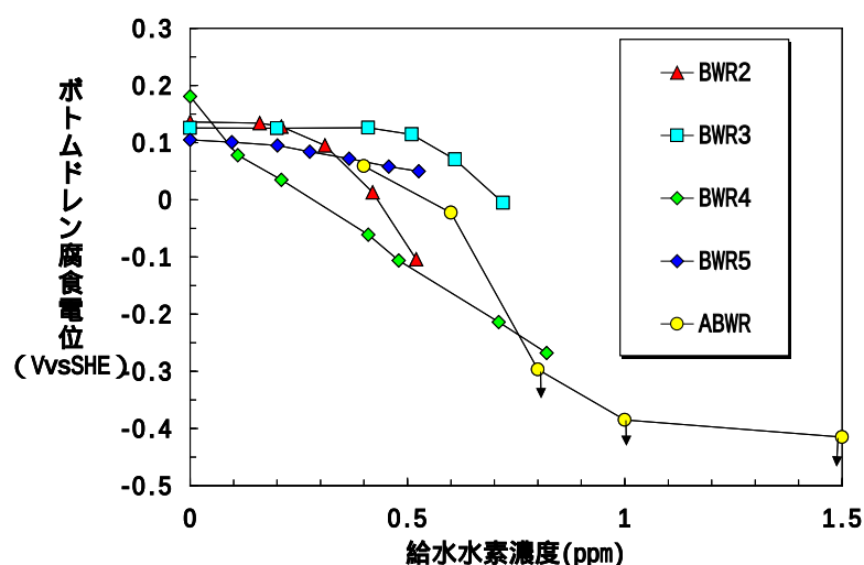
図 2.6 ボトムドレンの腐食電位と水素注入量との相関（実機での測定例） (4)
