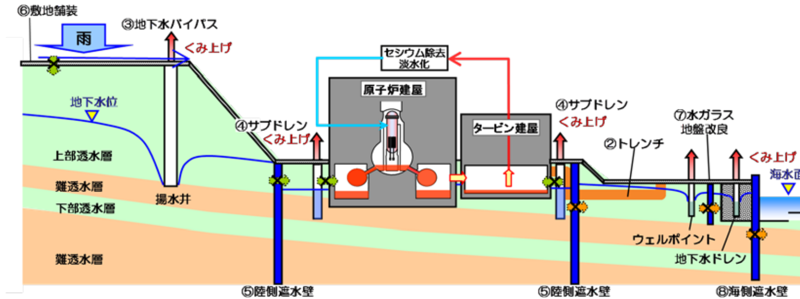
図 8.2-1 福島第一原子力発電所の汚染水対策の概要 [8.2-1]
