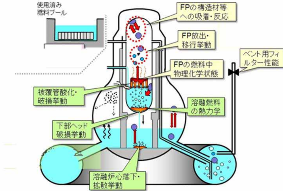
図 8.1-1 沸騰水型原子炉における SA 時の FP 挙動の模式図 [8.1-1]
