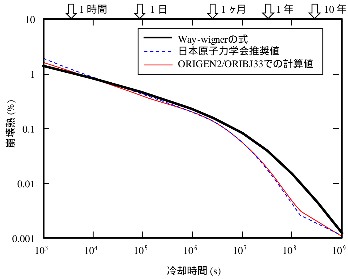
図 7.1.2-2 崩壊熱
