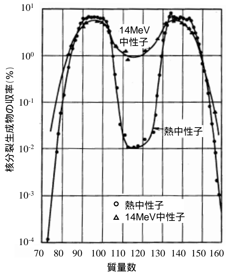
図 7.1.2-1 核分裂生成物の収率
