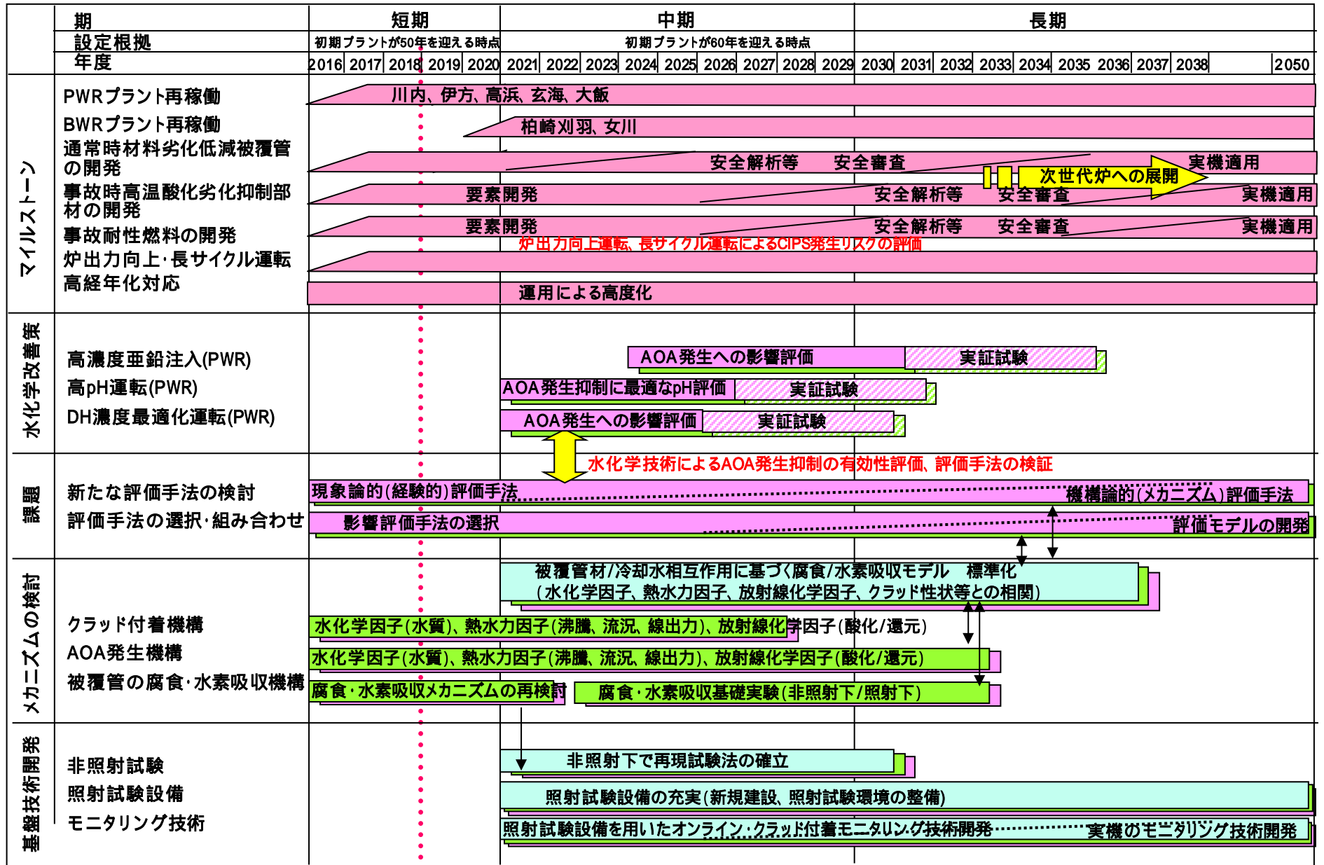
図 6.2.2-2 CIPS 対策による核燃料の性能維持のロードマップ
